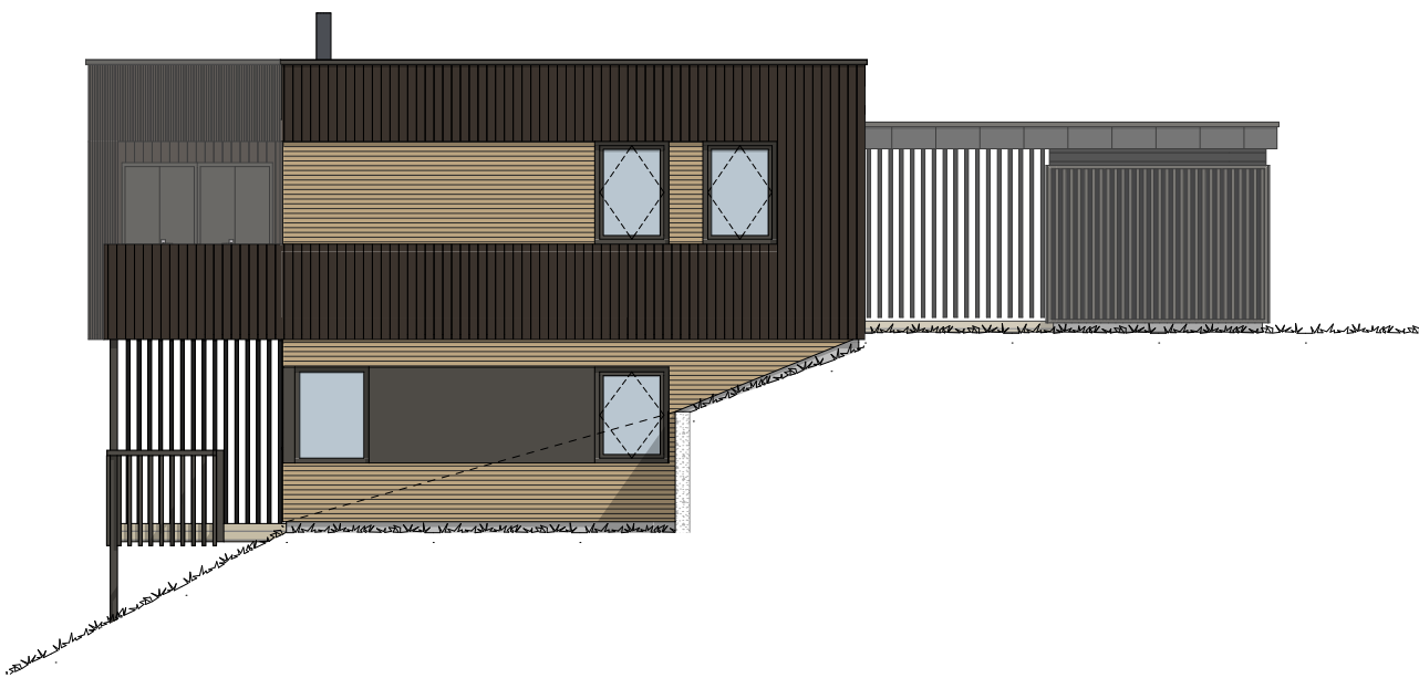
Fasade Sør
